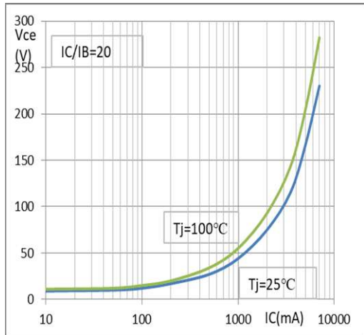
V_{CE(sat)} - I_C
