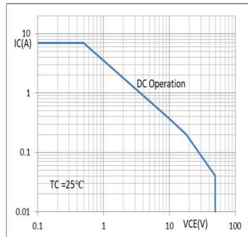
SOA
