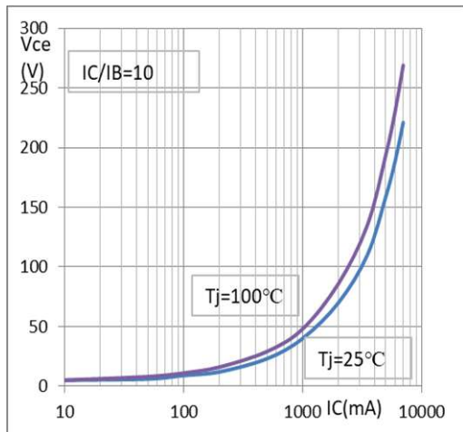
V_{CE(sat)} - I_C
